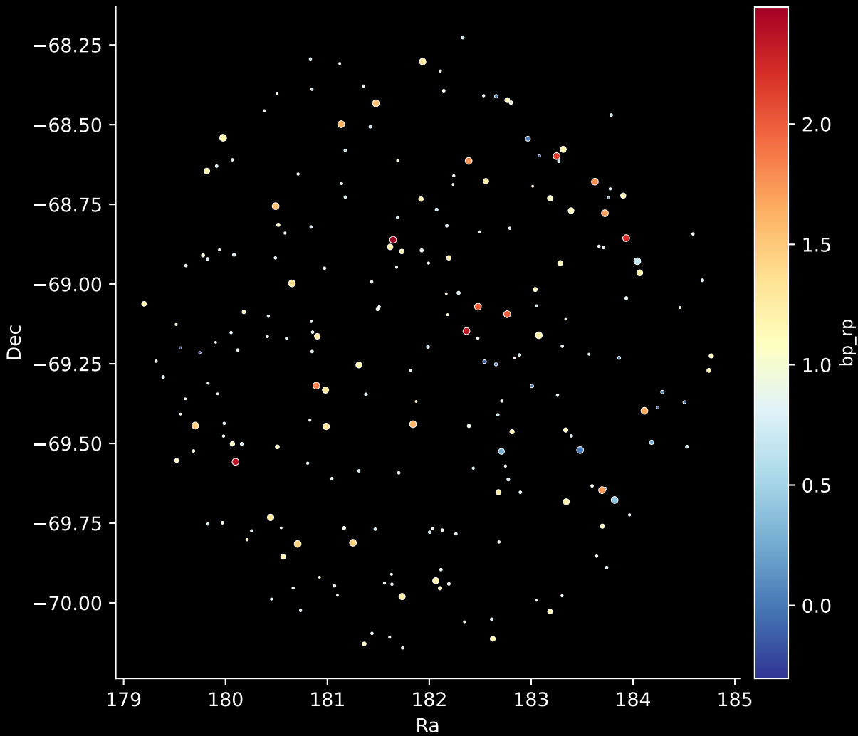
GALAH DR4 Field: [7135] Stars: 216
