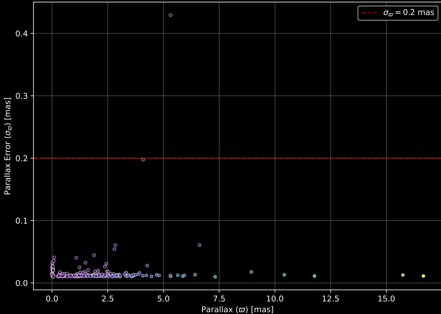
GALAH DR4 Field: [7135] Parallax Quality (n= 216)
