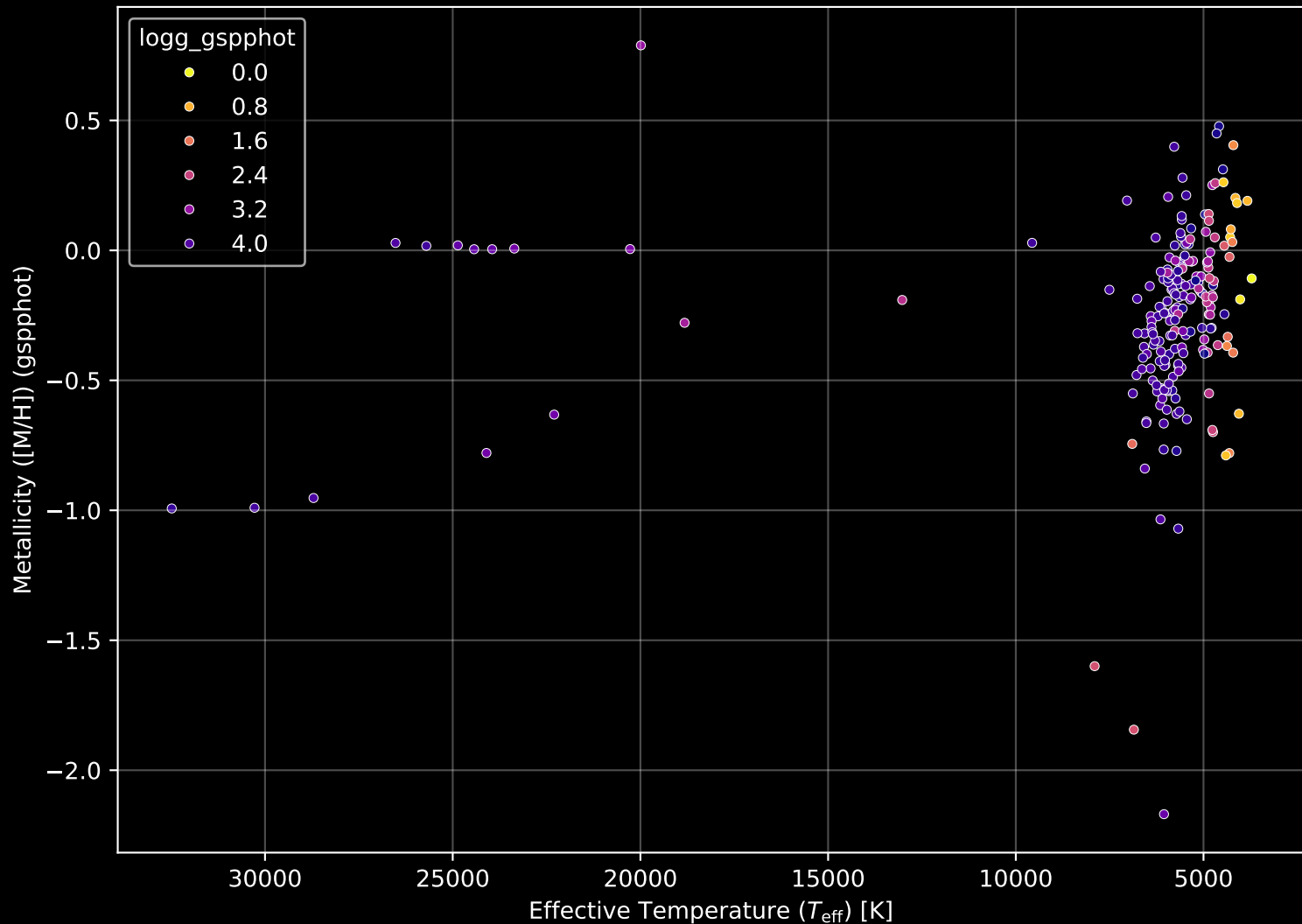
GALAH DR4 Field: [7135] Stellar Population Parameters (n= 216)
